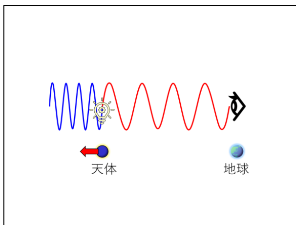
図5 ドップラーシフトによる赤方偏移（ビッグバン理論における赤方偏移）
