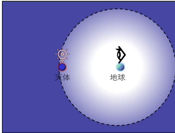
図6 拡張型ブラックホール宇宙モデルにおける赤方偏移のイメージ
