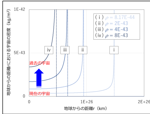
図7 拡張型ブラックホール宇宙モデルにおける宇宙の密度分布
