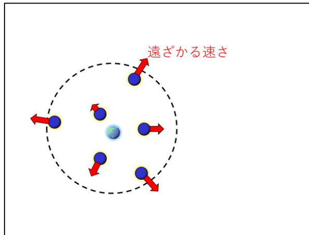
図4 地球から遠ざかる天体 (ハッブルの法則)
