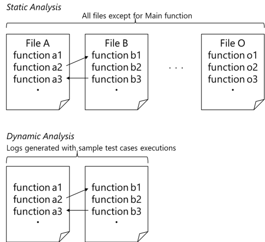
図 2 IoT サービスのプログラム自動分割時の分析
